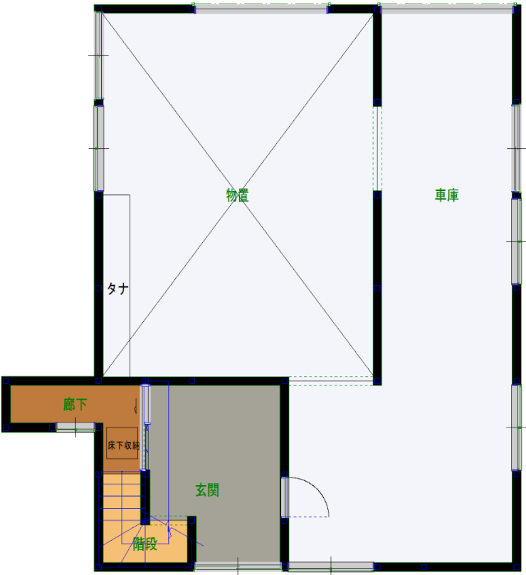
1 階平面図
