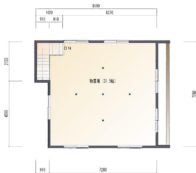
2階 平面図
