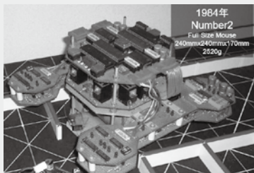
図1 33年前のマイクロマウス機体（森永氏）
