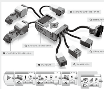
図5 レゴマインドストーム基本構成
