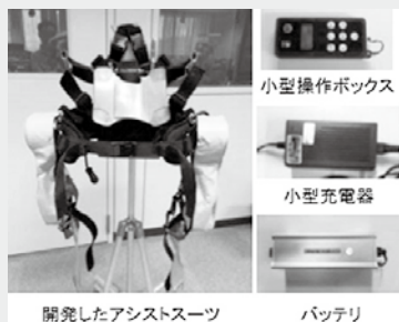
図1 農水省HPより 農業用アシストスーツ
