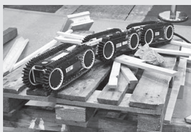
図4 ヘビ型瓦礫内探査 ロボット蒼竜
