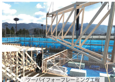
ツープайフォーフレーミング工程
