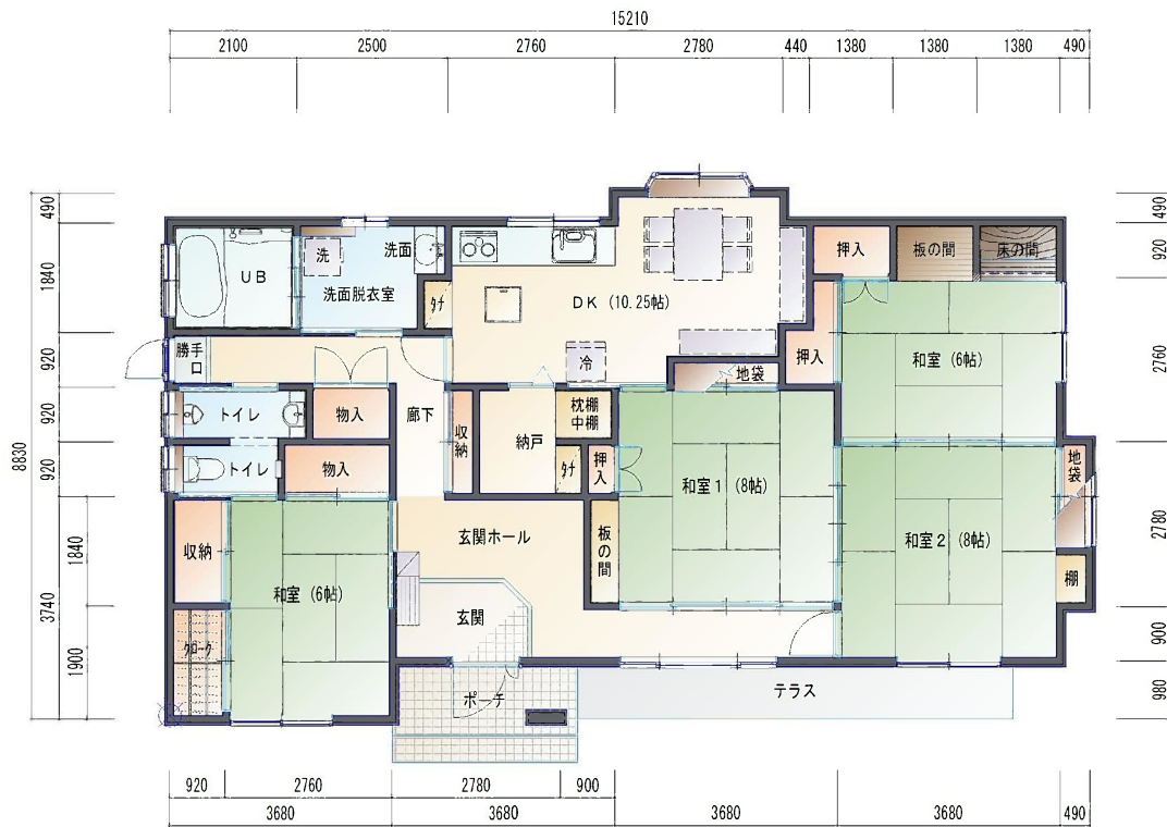
1階 平面図
