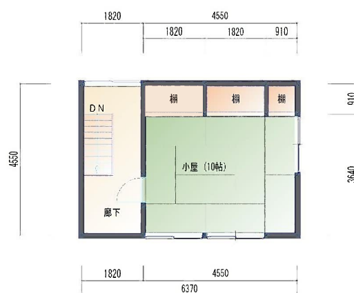
小屋 2階
