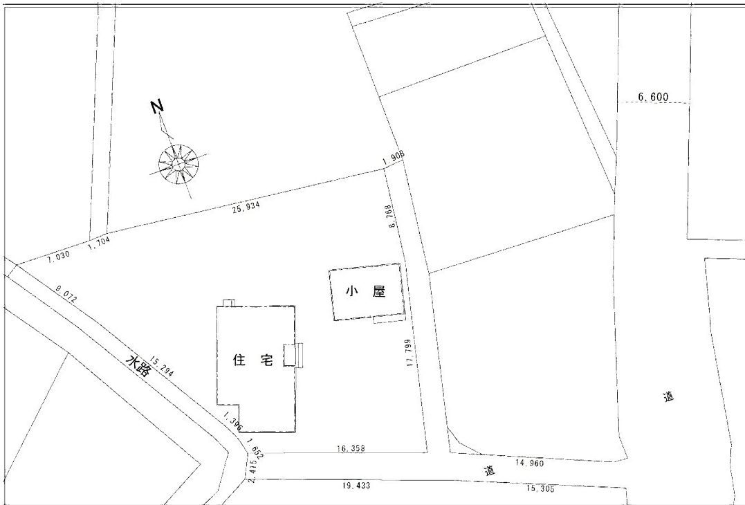
配置図
