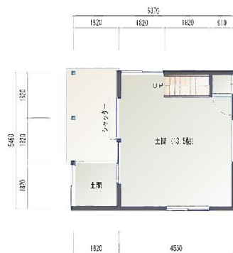
物置1階 平面図
