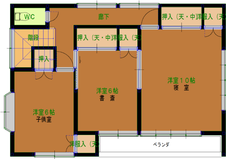
2 階平面図
