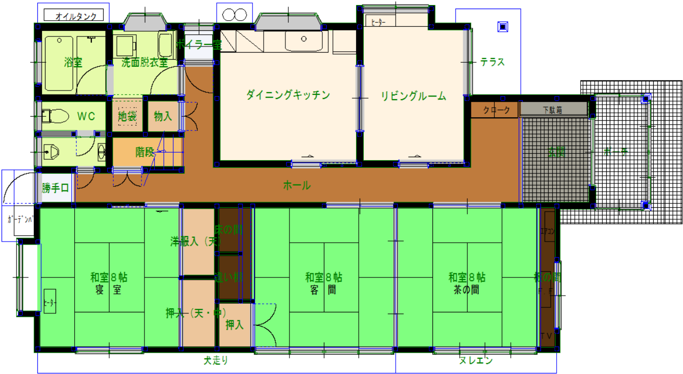
1 階平面図
