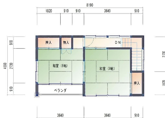
2階 平面図
