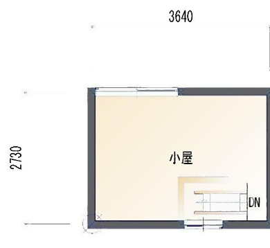
2階 平面図
