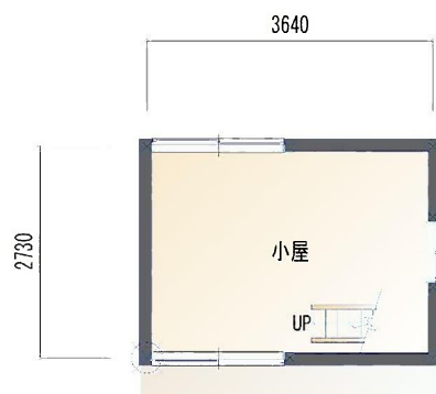
2階 平面図
