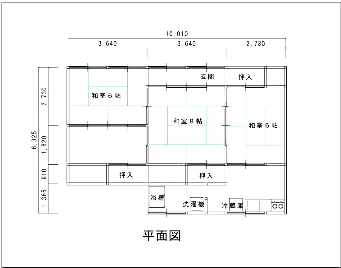
参考配置図
