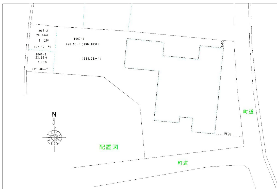
配 置 図
