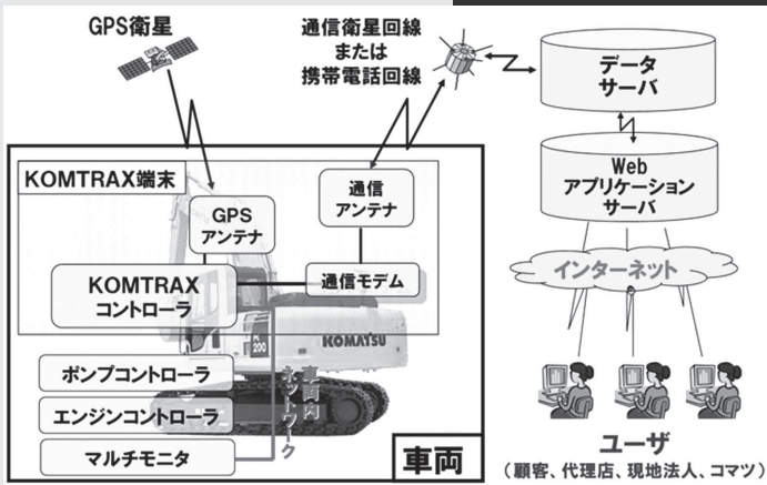
図2 建設機械遠隔操作モニタリングシステム(コマツ)
