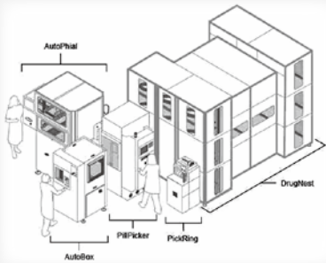
図2 自動薬剤管理ロボット 「pillpick」
