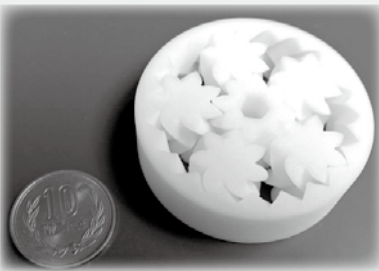
図1 分解できない遊星ギヤ 3Dプリンタで製作
