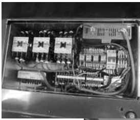
ソーラーユニット コントローラー
