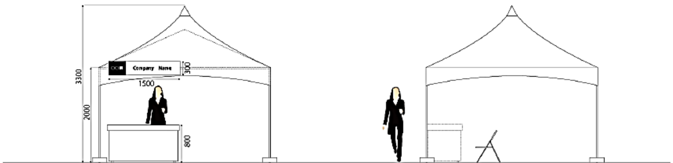
●立面図
